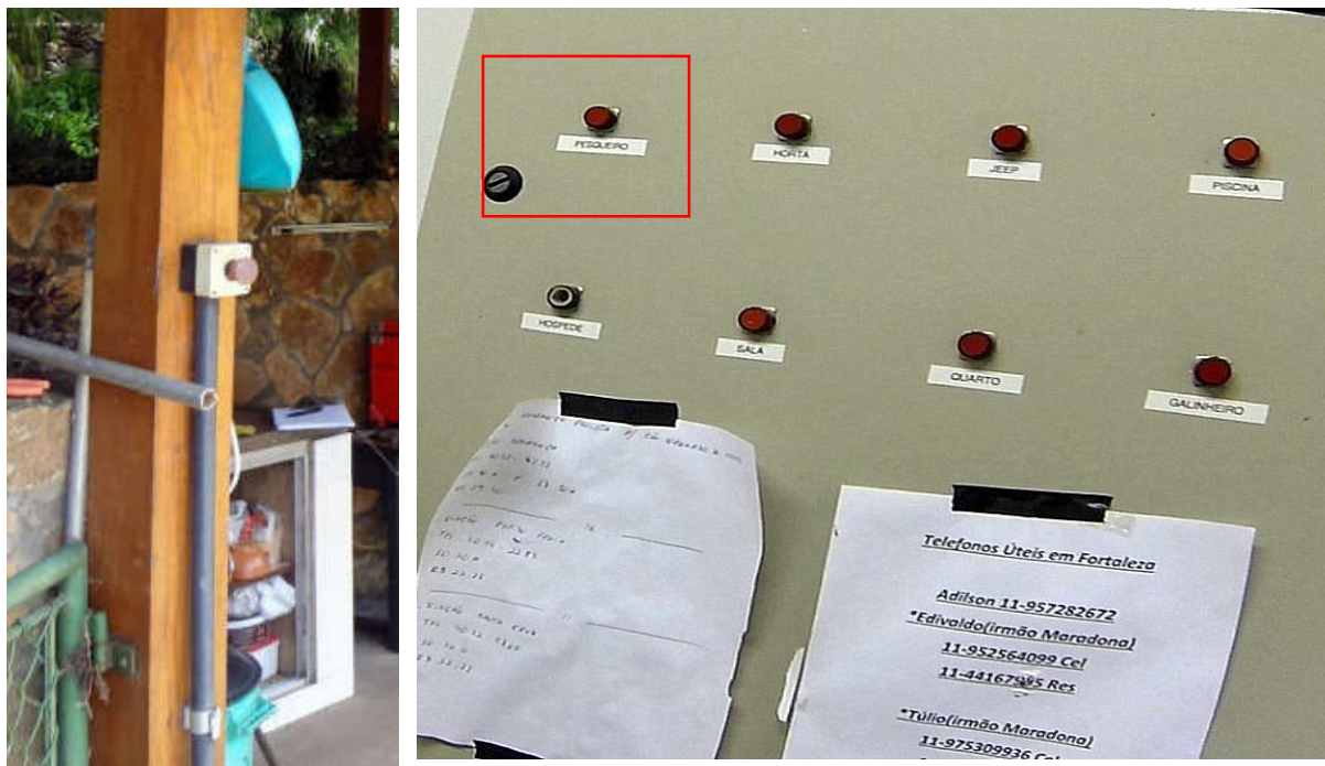
Figuras 85 e 86 – Botoeira de alarme instalada na área do Pesqueiro e painel no Alojamento dos Seguranças (em destaque indicador subtítulo “PESQUEIRO”).
